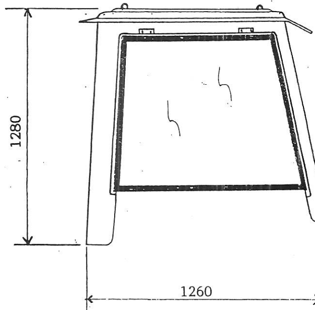
VUE COTE
