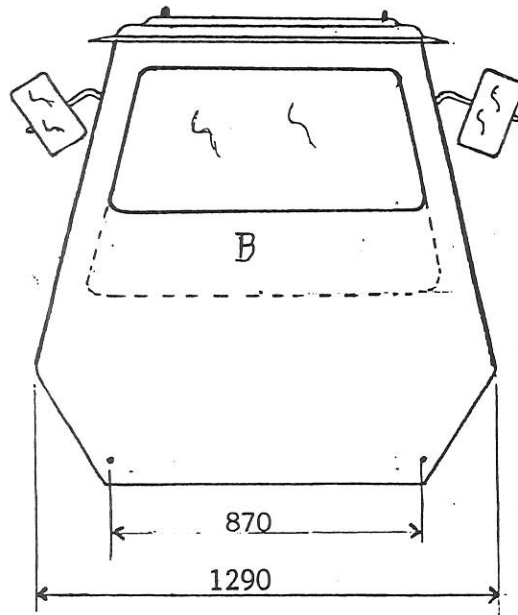
VUE ARRIERE
